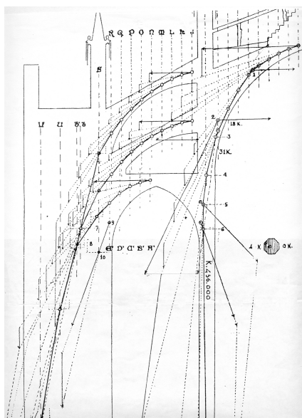
FIGURA 4. Càlcul gràfic de l'estructura de la catedral de Mallorca realitzat per Rubió i Bellver (fragment). (Font: J. Rubió, «Conferència sobre els conceptes orgànics, mecànics i constructius de la catedral de Mallorca», a Anuario , 1912.)
