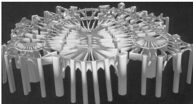
FIGURA 8. Model de l'estructura de la cripta de l'església de la Colònia Güell elaborat per a l'anàlisi de resistència mitjançant aplicacions informàtiques. (Fotografia de l'autor, 1996.)
